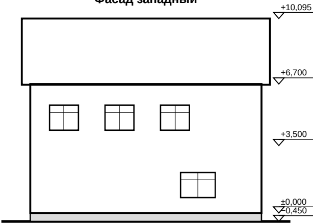
Фасад западный
