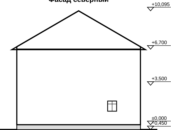
Фасад северный
