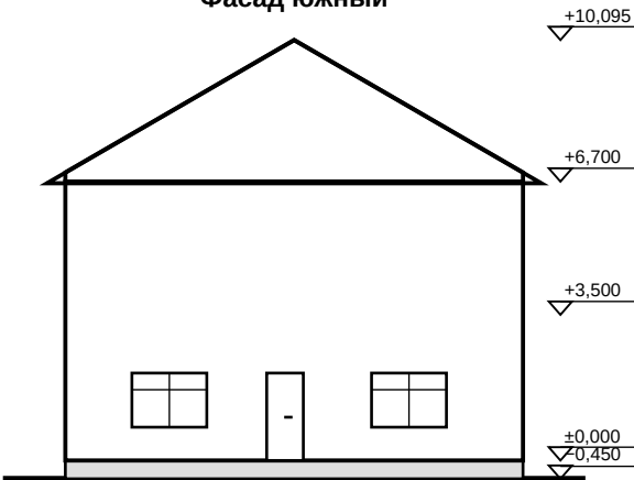
Фасад южный
