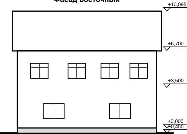
Фасад восточный
